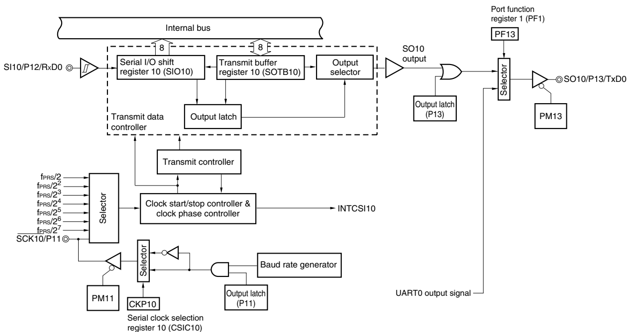
(b) 78K0/LF3
